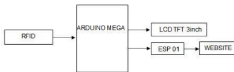
Gambar 2. 1 Diagram Blok Sistem Alat absensi mahasiswa berbasis website.
