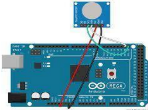
Gambar 2.4 Rangkaian RTC
