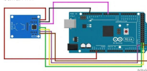
Gambar 2. 3 Rangkaian RFID pada arduino mega
