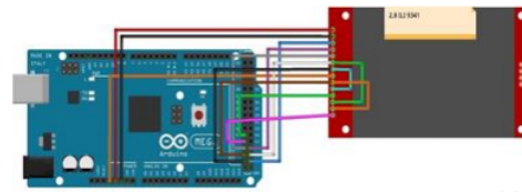
Gambar 2. 2 Rangkaian TFT
