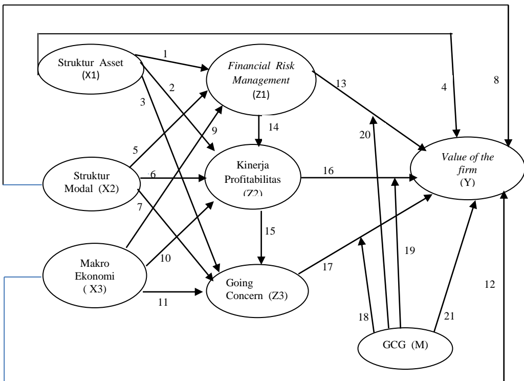
Gambar 3.2. Kerangka Konseptual
