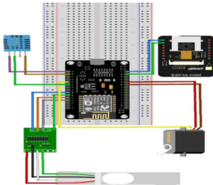
Gambar 3.3 Skematik alat
