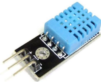
Gambar 2.6 DHT 11
