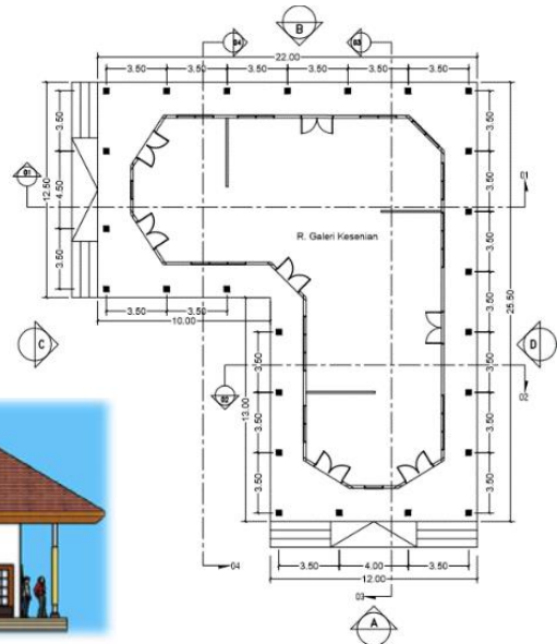
DENAH RUANG GALERI KESENIAN Skala 1:125
