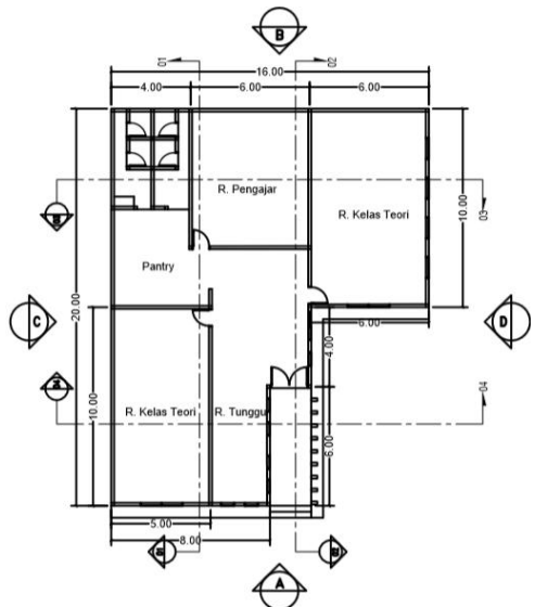
DENAH RUANG TEORI Skala 1:125
