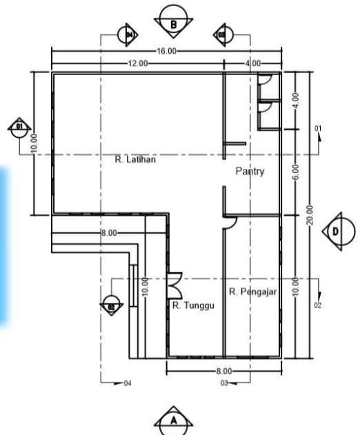
DENAH RUANG PELATIHAN Skala 1:125
