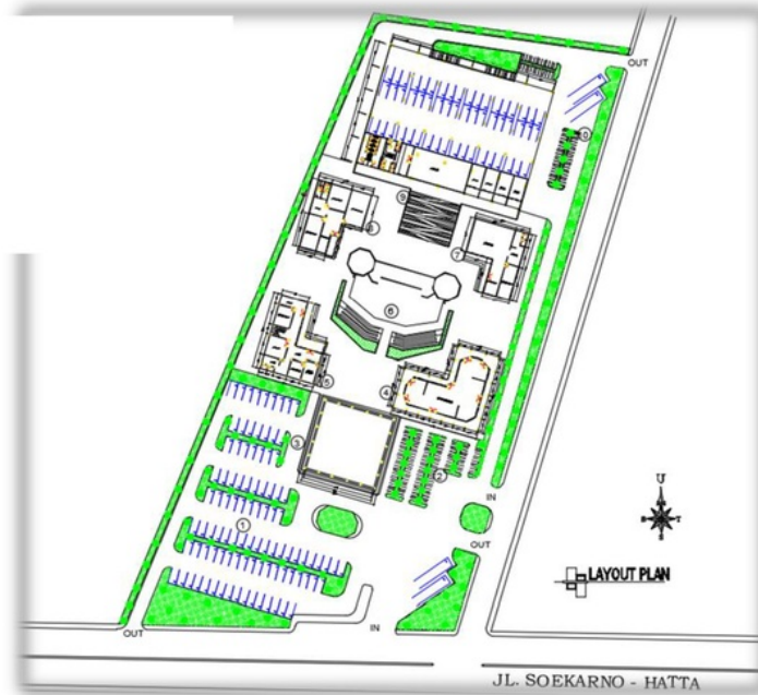
Gambar.3.10 Layout Plan Kawasan
