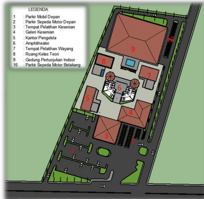
Gambar.3.11 Site Plan Kawasan
