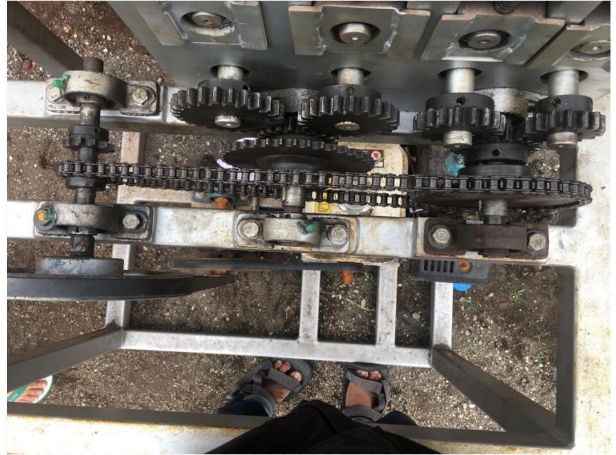
Pandangan samping mesin tebu
