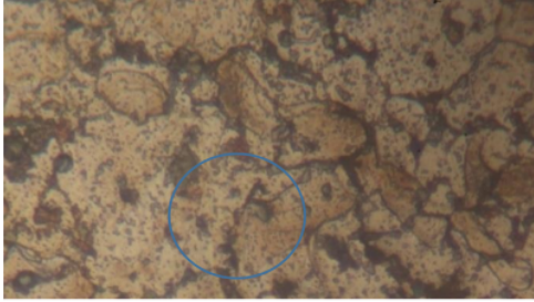
Gambar 4.21 struktur bainit
