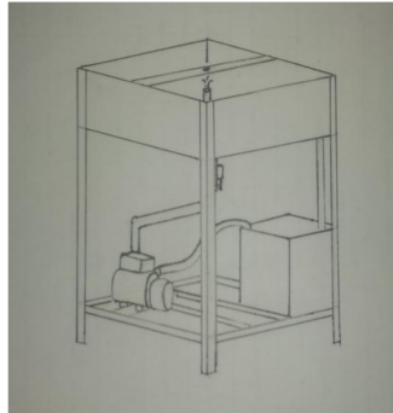
Gambar 3.1 desain alat
