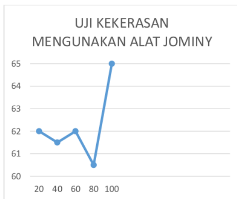
Gambar 4.15 grafik uji kekerasan menggunakan jominy test
