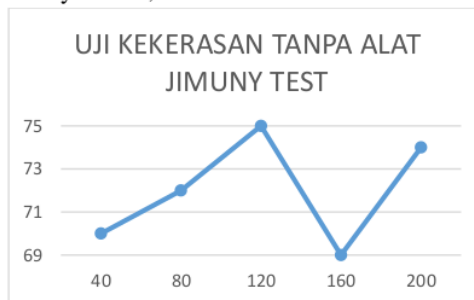
Gambar 4.16 grafik uji kekerasan tanpa pendinginan cepat
