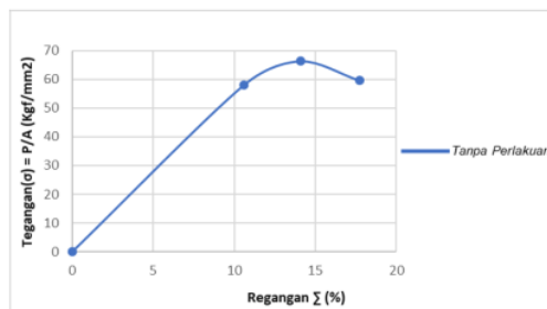
Grafik 1. Tegangan Regangan Baja ST 37 Tanpa Pengelasan
