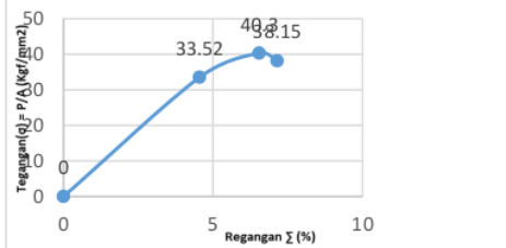
Grafik 5. Grafik Tegangan Regangan Baja ST37 dan ST42 dengan variasi putaran 880 Rpm dan waktu 30 detik
