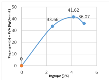
Grafik 3. Grafik Tegangan Regangan Baja ST37 dan ST42 dengan variasi putaran 1500 Rpm dan waktu 30 detik
