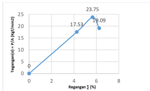
Grafik 7. Grafik Tegangan Regangan Baja ST37 dan ST42 dengan variasi putaran 1000 Rpm dan waktu 20 detik
