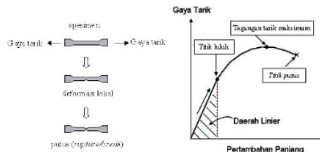
Gambar 3. Konsep Uji Tarik
