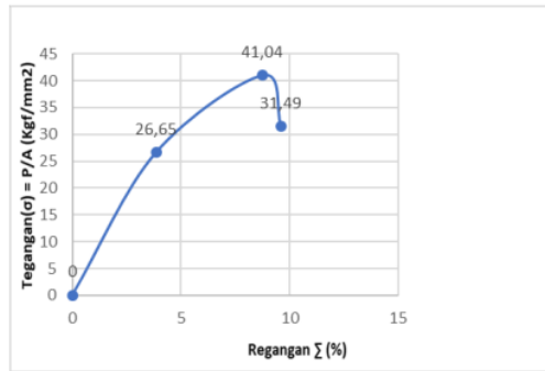
Grafik 4. Grafik Tegangan Regangan Baja ST37 dan ST42 dengan variasi putaran 1000 Rpm dan waktu 30 detik
