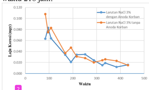
Gambar 4. 11 Grafik Laju Korosi Larutan NaCl 3%
