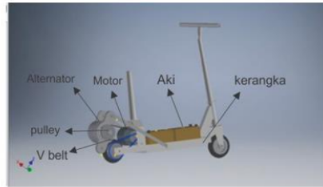
Gambar 3.1 Skuter dan Komponennya
