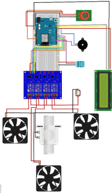
Gambar 3 Diagram Pengkabelan
