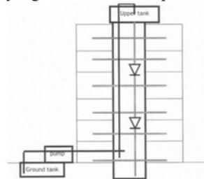
Gb.6.. Konsep penyediaan air bersih. Sumber:internet
