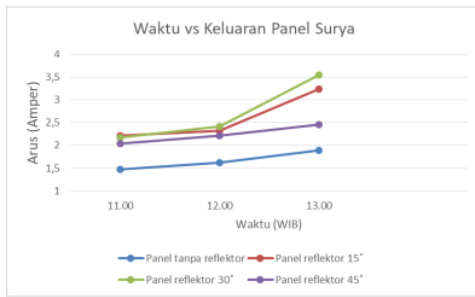
Gambar 10. Grafik keluaran arus panel surya menggunakan reflektor cermin C dan tanpa menggunakan reflektor cermin
