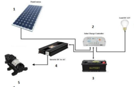
Gambar 4. Komponen sistem pembangkit listrik energi surya
