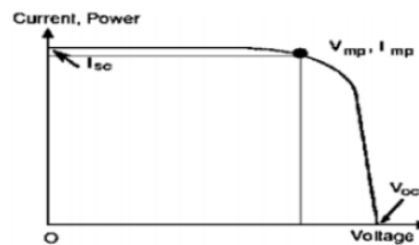
Gambar 1. Kurva karakteristik V - I
