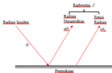
Gambar 2. Radiositas
