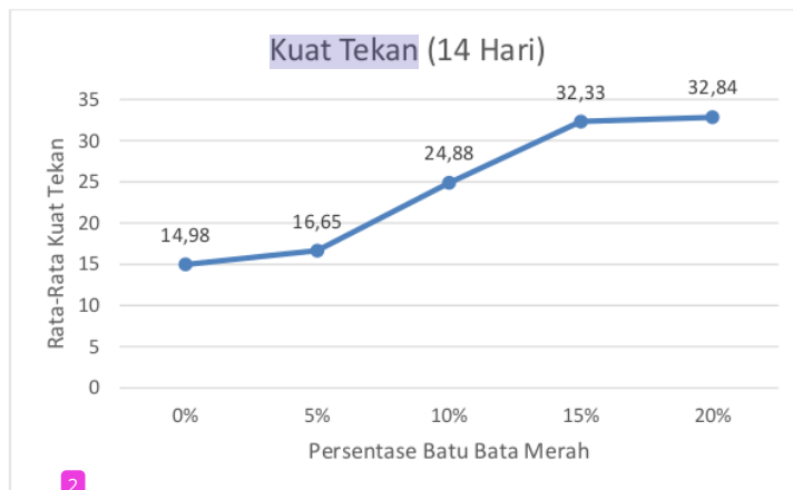
2 Gambar 4.27 Grafik Kuat Tekan Beton Alir Umur 14 Hari
