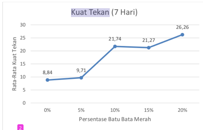
2 Gambar 4.26 Grafik Kuat Tekan Beton Alir Umur 7 Hari
