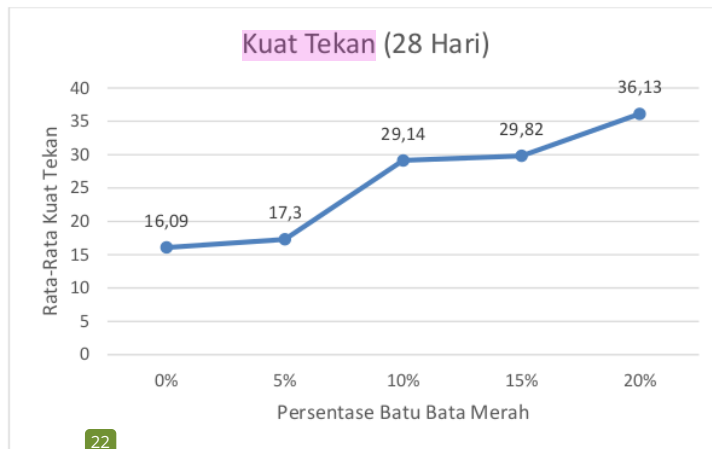
Gambar 4.28 Grafik Kuat Tekan Beton Alir Umur 28 Hari
