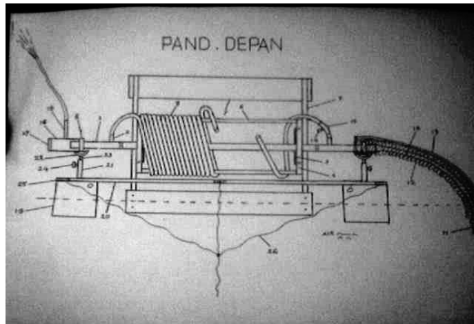
Desain Gambar pandangan depan Pompa hydam Spiral
