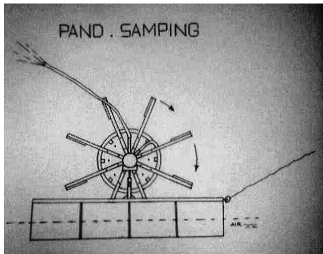
Desain Gambar pandangan samping Pompa hydam Spiral
