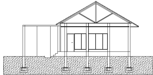
POTONGAN B
