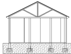
POTONGAN A
