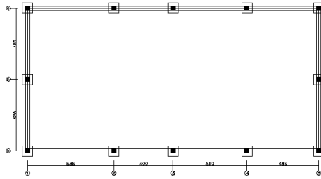
RENCANA PONDASI DAN SLOF
