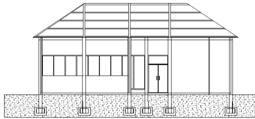
POTONGAN B
