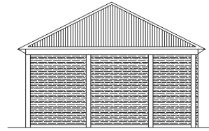
TAMPAK TIMUR
