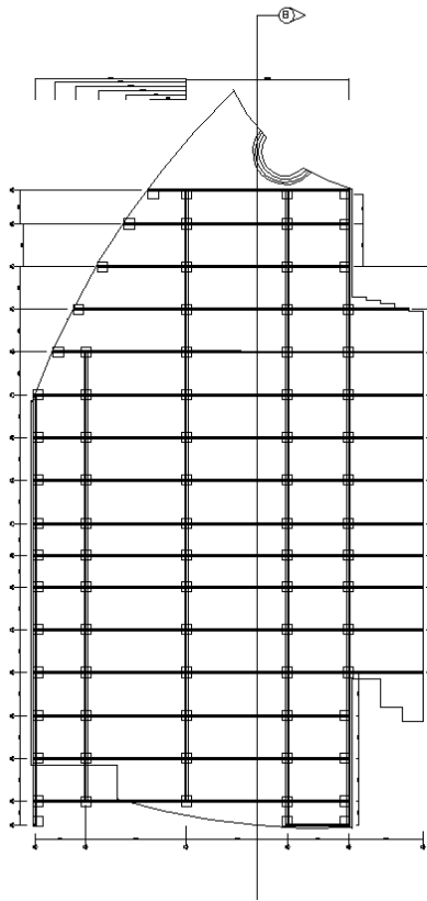
Rencana Massa 1 dan 3
