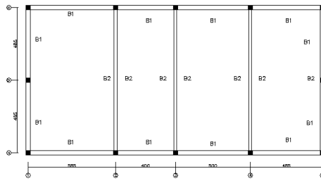
RENCANA BALOK
