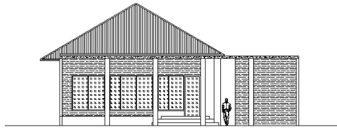
TAMPAK SELATAN
