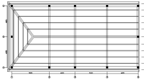
RENCANA ATAP
