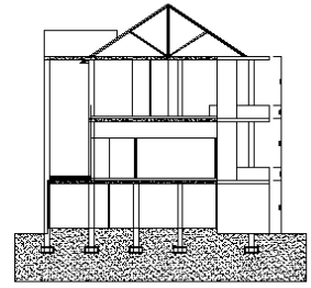
POTONGAN B-B
