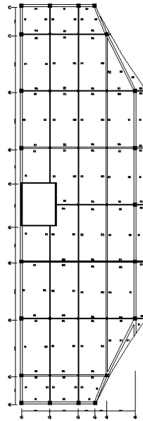
RENCANA BALOK
