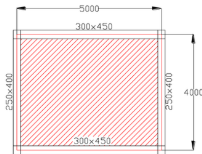
Gambar 1.1 Desain Pelat Lantai
