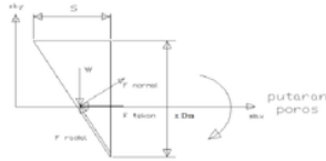
Gambar 2.2 Penjelasan arah gaya
