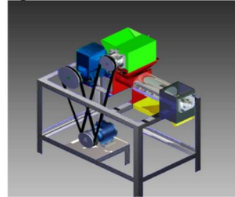
Gambar 2.1 Desain 3D Rangkaian Mesin
