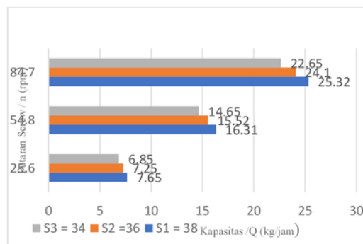
Gambar Grafik Hasil Pengujian Pengaruh Putarandan Jarak Pitch Screw Terhadap Kapasitas
