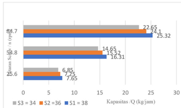
Gambar Grafik Hasil Pengujian Pengaruh Putarandan Jarak Pitch Screw Terhadap Kapasitas
