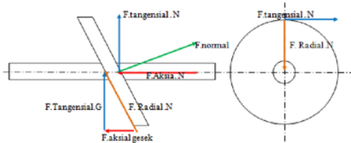
Gambar 2.3 Gaya yang terjadi pada screw
