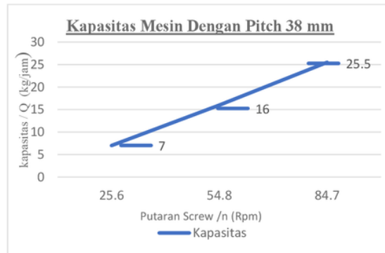
Gambar Grafik Pengujian pengaruh putaran dengan jarak pitch screw 38 mm
