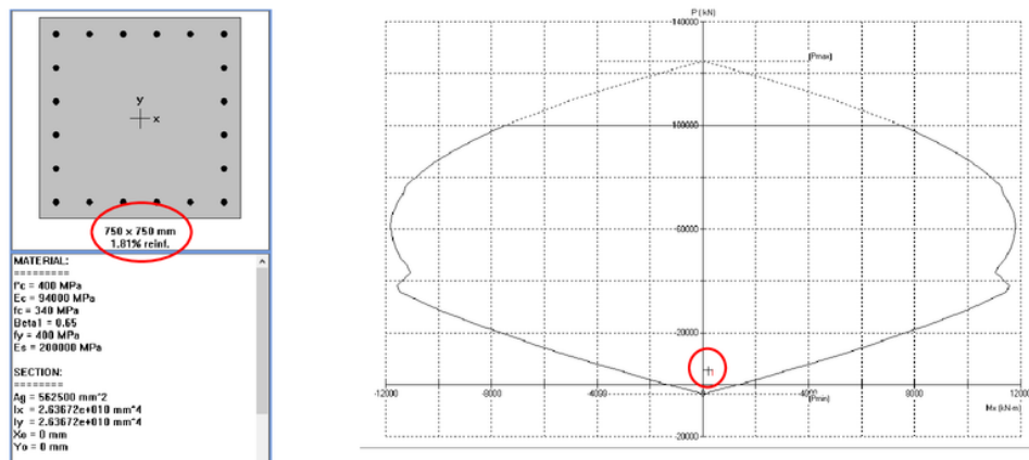
Gambar 4.5 Presentase tulangan kolom lantai 3 & Diagram interaksi aksial vs momen kolom
