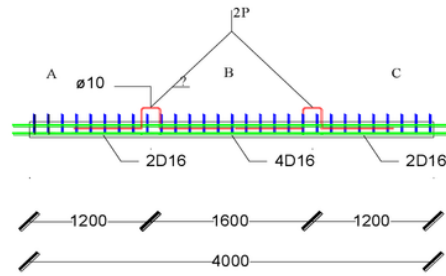
Gambar 4.4 Letak titik pengangkatan balok (AutoCad 2017)
