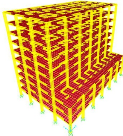
Gambar 4.1. Pemodelan Gedung (permodelan SAP 2000 V.19)
