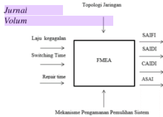
Gambar 1. Skema FMEA
