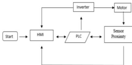
Gambar 3.2 Blok Diagram
