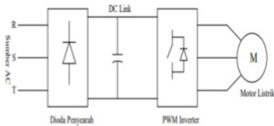
Gambar 2.3 Bagian utama inverter
