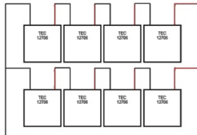
Gambar 3.3 TEG menggunakan rangkaian Seri Paralel (Campuran)
