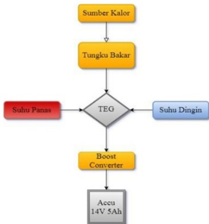
Gambar 3.6 Blok Diagram Rancangan Sistem Penelitian
