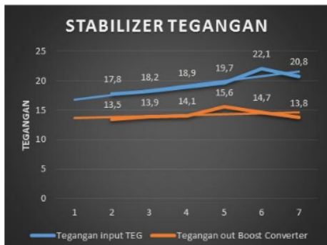
Gambar 4.13 Grafik Tegangan keluaran TEG ke Buck Boost Converter
