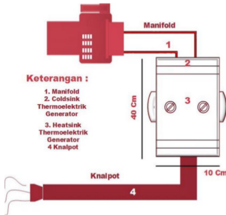
Gambar 4 : Desain Alat
