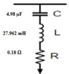
Gambar 2. Rangkaian Desain Filter Pada SDP 2 Phasa R Orde 3
