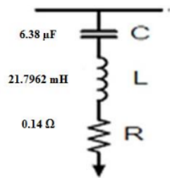
Gambar 3. Rangkaian Desain Filter Pada SDP 2 Phasa S Orde 3
