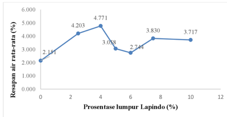
Gambar 4.10 Grafik Resapan Air Rata-rata (Sumber : Penulis)
