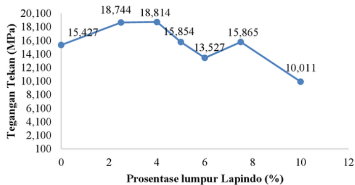
Gambar 4.8 Grafik Tegangan Tekan (Sumber : Penulis)
