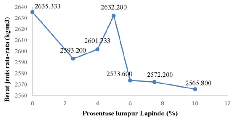
Gambar 4.9 Grafik Berat Jenis Rata-rata (Sumber : Penulis)
