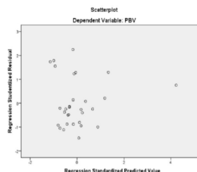
Gambar 4.1 Hasil Uji Heteroskedastisitas
