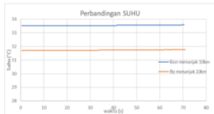
Gambar 4. 8 Perbandingan suhu jalur menanjak kecepatan 10km/jam
