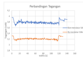
Gambar 4. 5 Perbandingan tegangan jalur mendatar kecepatan 50km/jam
