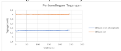
Gambar 4. 2 Perbandingan tegangan jalur mendatar kecepatan 10km/jam
