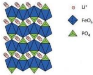
Gambar 2. 3 Struktur kristal dari LiFePO4 [8]
