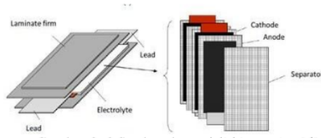
Gambar 2. 2 Struktur baterai lithium – ion [6]
