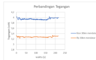
Gambar 4. 4 Perbandingan tegangan jalur mendatar kecepatan 30km/jam
