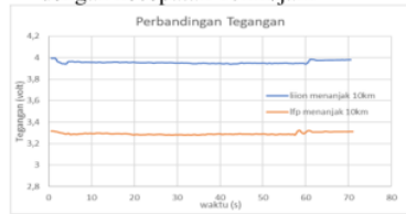
Gambar 4. 7 Perbandingan tegangan jalur menanjak kecepatan 10km/jam
