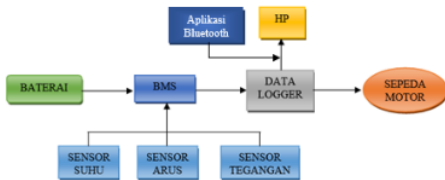
Gambar 2.4 Diagram Blog Pengujian Discharge
