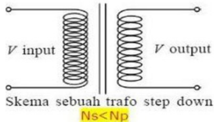
Gambar 5 Kumpulan Trafo Step Down
