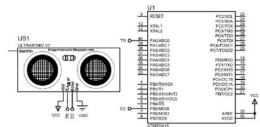
Gambar 8 Rangkaian Sensor Ultrasonik
