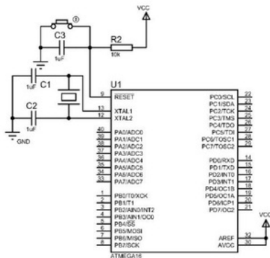
Gambar 9 Rangkaian Mikrokontroler
