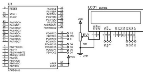
Gambar 10 Rangkaian LCD 2x16
