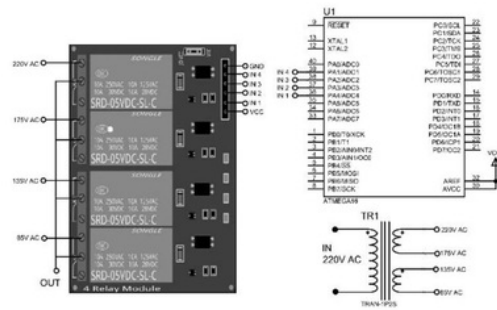
Gambar 11 Rangkaian Modul Relay
