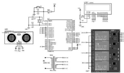
Gambar 7 Rangkaian Keseluruhan
