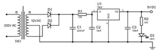
Gambar 12 Rangkaian Catu Daya
