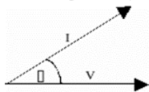
Gambar 2.3 Arus Tertinggal dari Tegangan Sebesar Sudut phi
