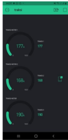
Gambar 4.1.2 Tampilan saat tanpa ada gangguan
