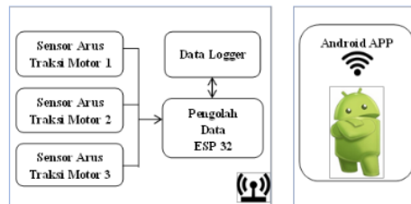
Gambar 3.1 Blok Diagram Aplikasi Monitoring Arus
