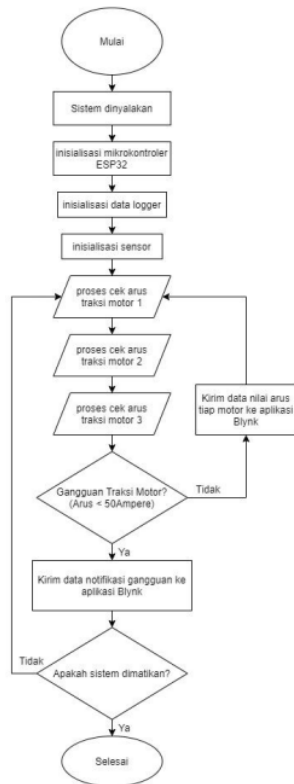
Gambar 3.2 Flowchart sistem keseluruhan
