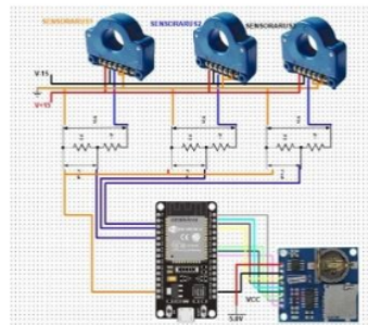
Gambar 3.1.1 Skematik Sistem
