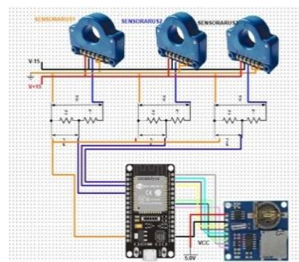
Gambar 3.1.1 Skematik Sistem
