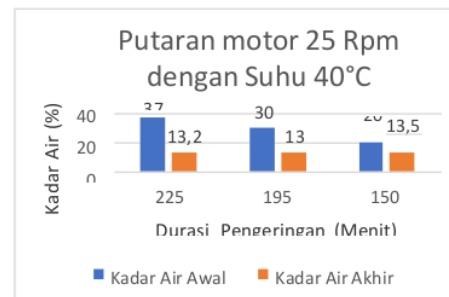
Gambar 9 grafik Putaran motor 25 Rpm dengan Suhu 40°C
