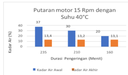
Gambar 12 grafik Putaran motor 15 Rpm dengan Suhu 40°C
