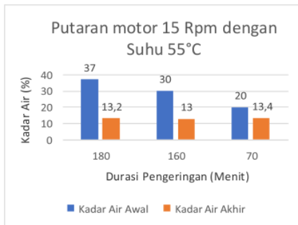
Gambar 14 grafik Putaran motor 15 Rpm dengan Suhu 55°C
