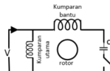
Gambar 3 motor satu fasa
