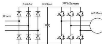
Gambar 2 skema VFD untuk mengatur kecepatan motor
