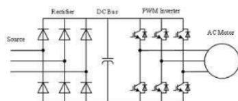
Gambar 4 skema VFD untuk mengatur kecepatan motor
