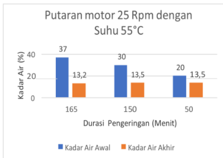
Gambar 11 grafik Putaran motor 25 Rpm dengan Suhu 55°C
