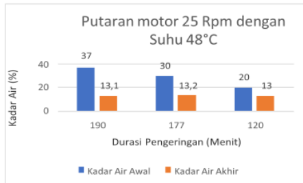
Gambar 10 grafik Putaran motor 25 Rpm dengan Suhu 48°C
