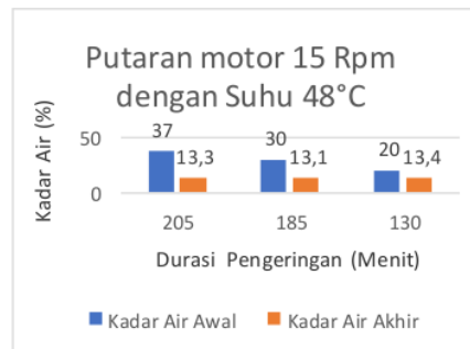
Gambar 13 grafik Putaran motor 15 Rpm dengan Suhu 48°C
