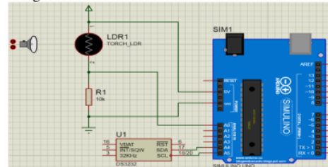
Gambar 3. 3 Rangkaian RTC dan sensor LDR
