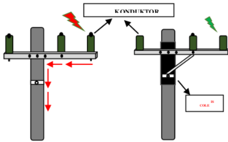
Gambar 3.5 Ilustrasi cara kerja ISCOLE
