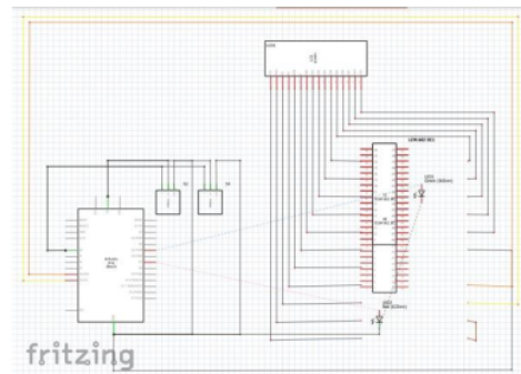
Gambar 3.3 Layout Rangkaian Keseluruhan dalam Bentuk Fritzing
