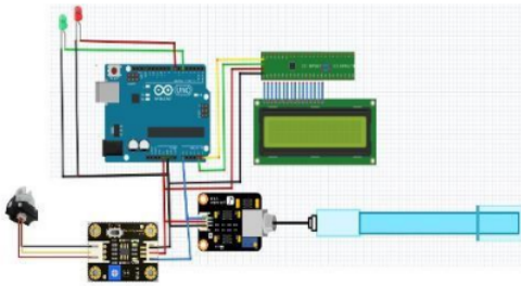
Gambar 3.4 Layout Rangkaian Keseluruhan Dalam Bentuk Gambar
