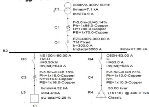
Gambar 2. Simulasi Perbaikan Faktor Daya
