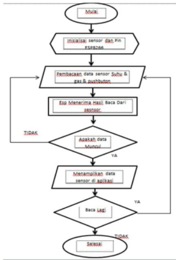
Gambar 3.5 Flowchart Pembacaan DHT11 & MQ135
