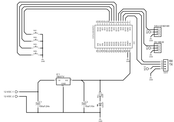
Gambar 3. Desain Skematik Rangkaian
