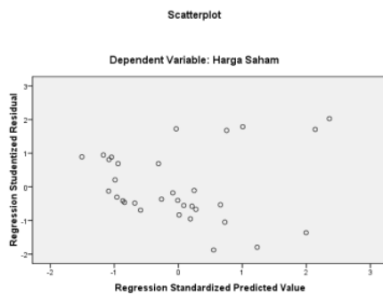
Gambar 4.1 Uji Heterokedastisitas
