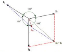
Gambar 6 Vektor Diagram Arus Tidak Seimbang
