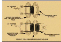
Gambar 1 Prinsip hukum elektromagnetik
