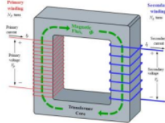
Gambar 2 Prinsip kerja transformator
