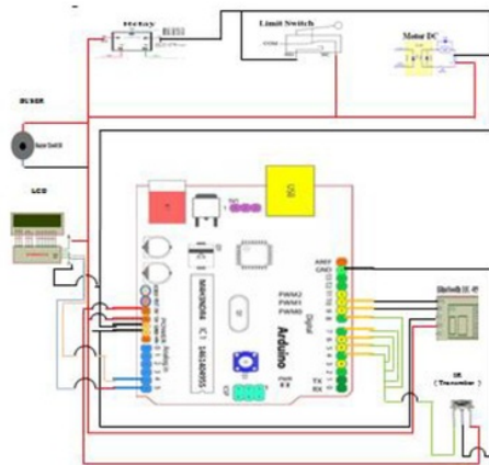
Gambar 3.6 Rangkaian Secara Detail
