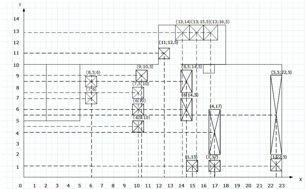
Gambar Blok layout awal
