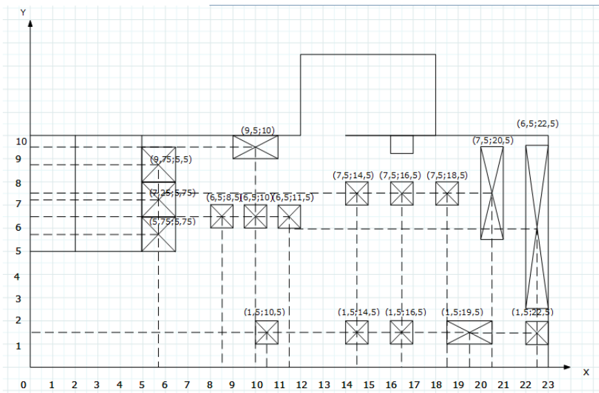
Gambar blok layout usulan
