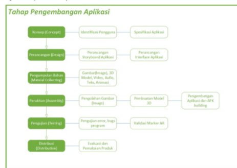
Gambar 1. Pengembangan Sistem
