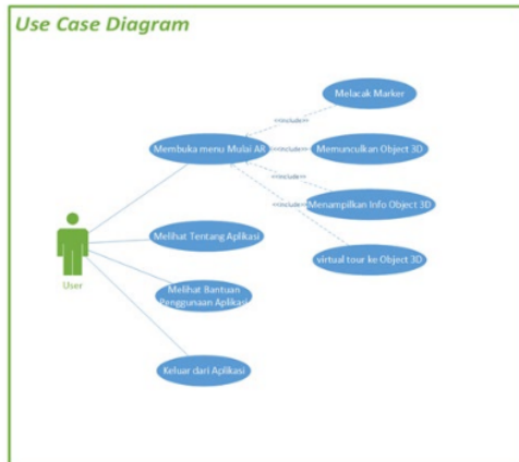
Gambar 2. Diagram Usecase Aplikasi
