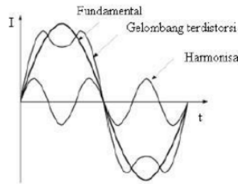
Gambar 1. Gelombang Fundamental dan Gelombang Harmonisa. [3]
