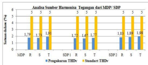
Gambar 6. Grafik Analisa Sumber Harmonisa Tegangan dari MDP/ SDP
