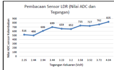
Gambar 4.2 Pembacaan Sensor LDR
