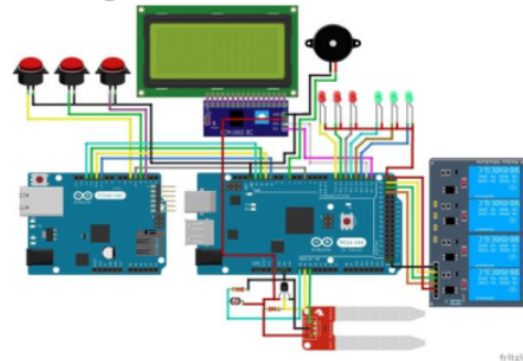
Gambar 3.2 Rangkaian Keseluruhan Sistem
