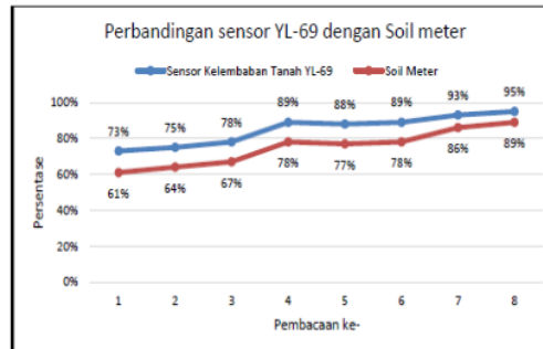
Gambar 4.3 Perbandingan sensor YL-69 dengan Soil Meter
