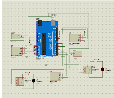
Gambar 1. Rangkaian sistem
