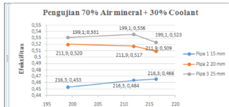
Grafik 4.9 Hubungan antara variasi diameter pipa terhadap efektifitas radiator komposisi fluida 30% Coolant + 70% Air mineral.
