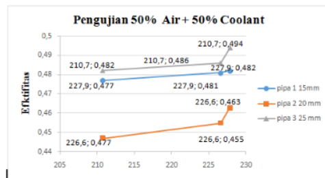
Grafik 4.1 Hubungan variasi diameter pipa dengan efektifitas radiator pada komposisi fluida 50% Coolant + 50% Air mineral.
