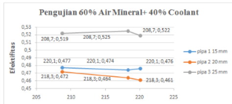
Grafik 4.8 Hubungan antara variasi pipa diameter dengan efektifitas radiator komposisi fluida 40% Coolant + 60% Air mineral.
