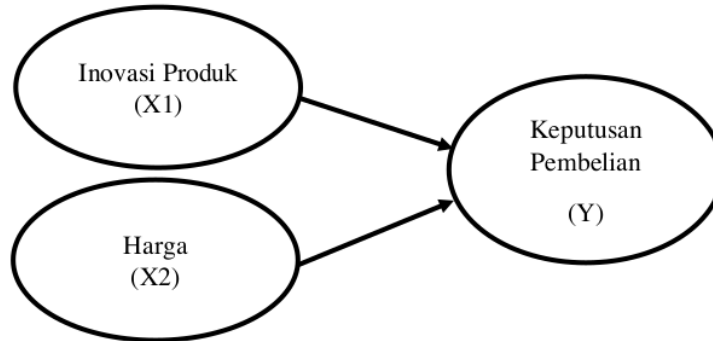
Gambar 1 Kerangka Pemikiran
