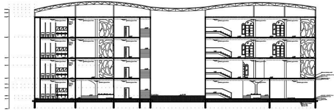
Potongan A-A Massa Edukasi
