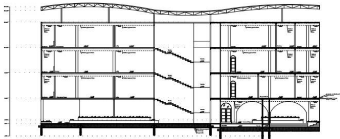
Potongan B-B Massa Pengelola
