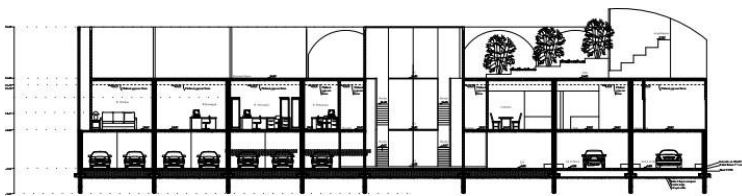
Potongan A-A Massa Pengelola
