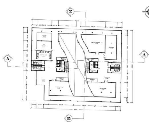
Denah Massa Edukasi Lt. 2
