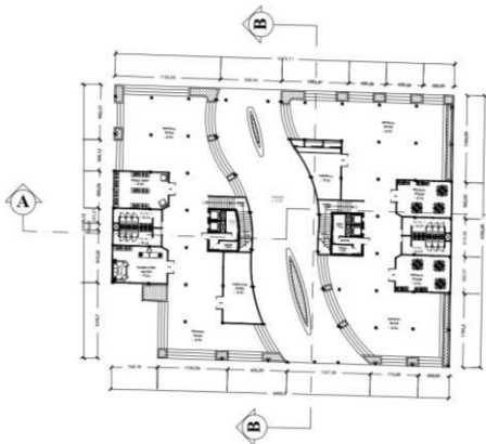
Denah Massa Edukasi Lt. 1
