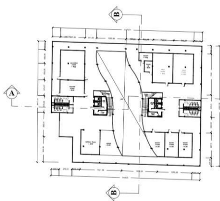
Denah Massa Edukasi Lt. 3
