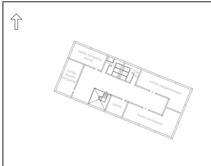
Lampiran 12. Denah Lantai 3 Massa Penunjang
